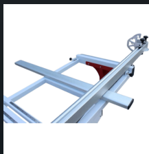
Στήριγμα πάνελ στον δικτυωτό βραχίονα
